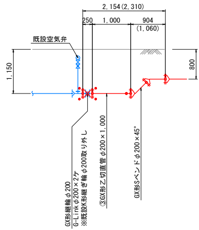
詳細図① S=1:50 (A1) 西南既設管接続部 S=1:100 (A3)
