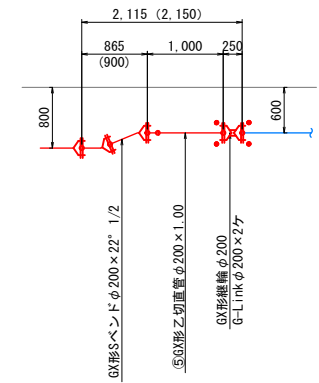
詳細図④ S=1:50 (A1) 東側既設管接続部 S=1:100 (A3)
