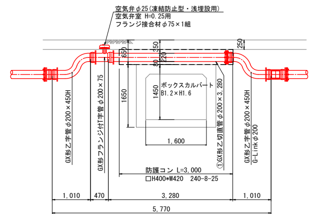
詳細図③ S=1:50 (A1) 空気弁設置箇所 S=1:100 (A3)
