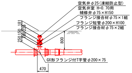
詳細図② S=1:50 (A1) 空気弁設置箇所 S=1:100 (A3)
