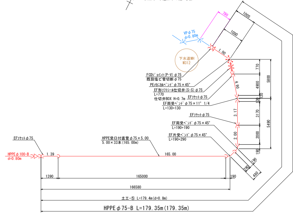
HPPE φ75-B
