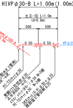
HIVP φ30-B
